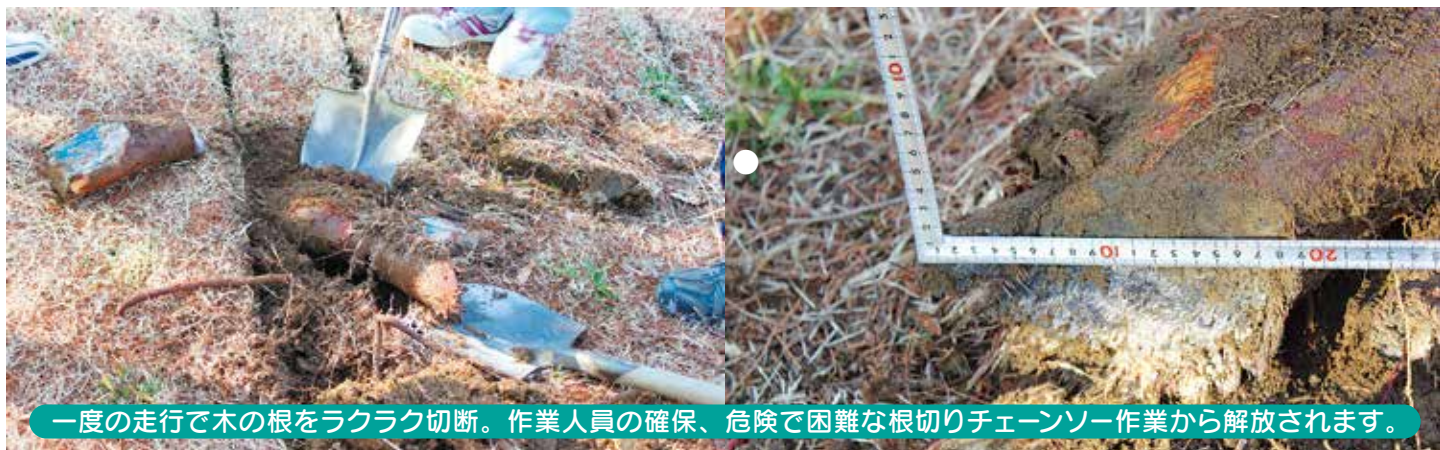
3枚×2列のプレートがしっかりと木の根を両側から切断
